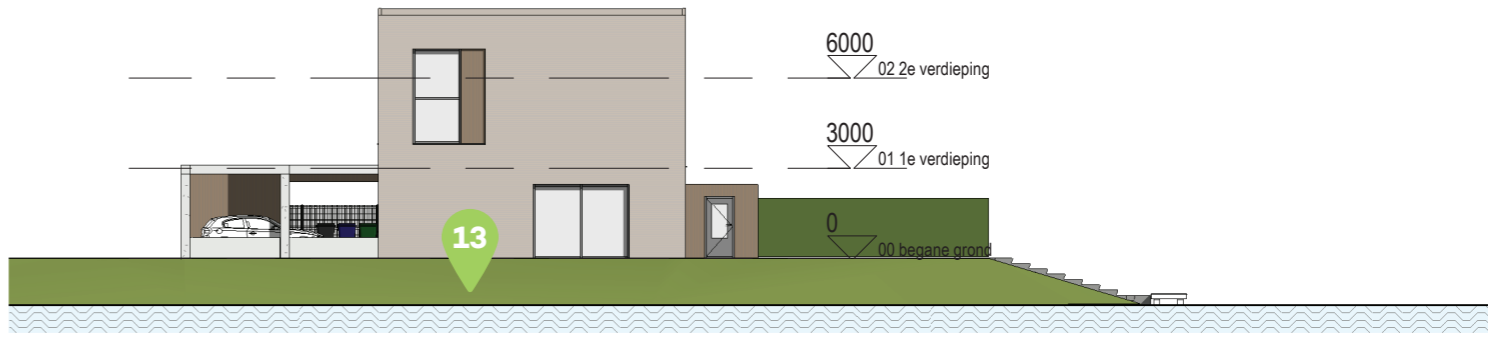
Rechter zijgevel
